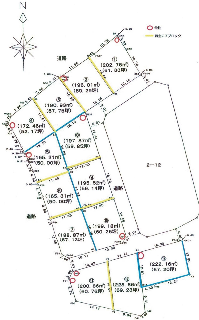
分筆計画図 S=1:500
